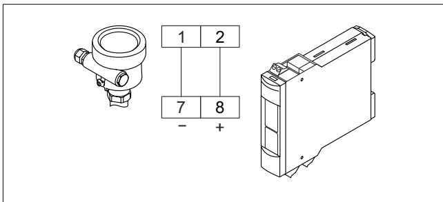
3 Povezava naprave s poljubnim senzorjem NAMUR
