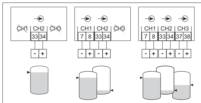
3 Tilslutning til alle NAMUR-sensorer for 1 til 3 grænse signaler
