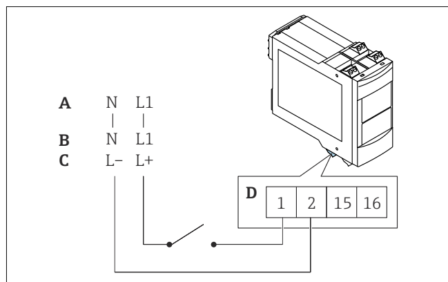
2 Расположение клемм питания
