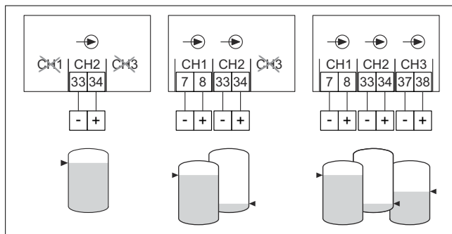
3 Подключение к любому датчику NAMUR для 1-3 предельных сигналов
