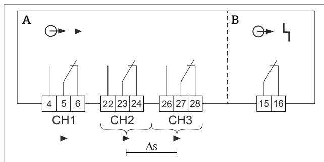
4 Подключение выходов
