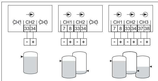
☐ 3 1~3개의 제한 신호를 위한 NAMUR 센서 연결
