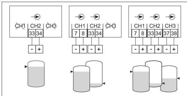
3 Collegamento a qualsiasi sensore NAMUR per 1 ... 3 segnali di soglia
