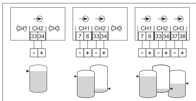
3 Conectarea la orice senzor NAMUR pentru 1 până la 3 semnale pentru valoare limită
