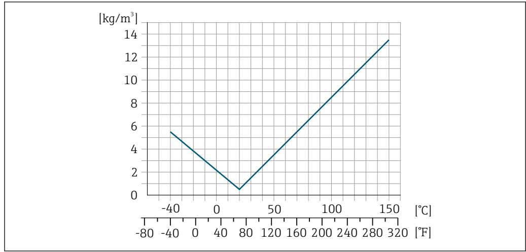
24 Felddichtejustierung, Beispiel bei +20 °C (+68 °F)
