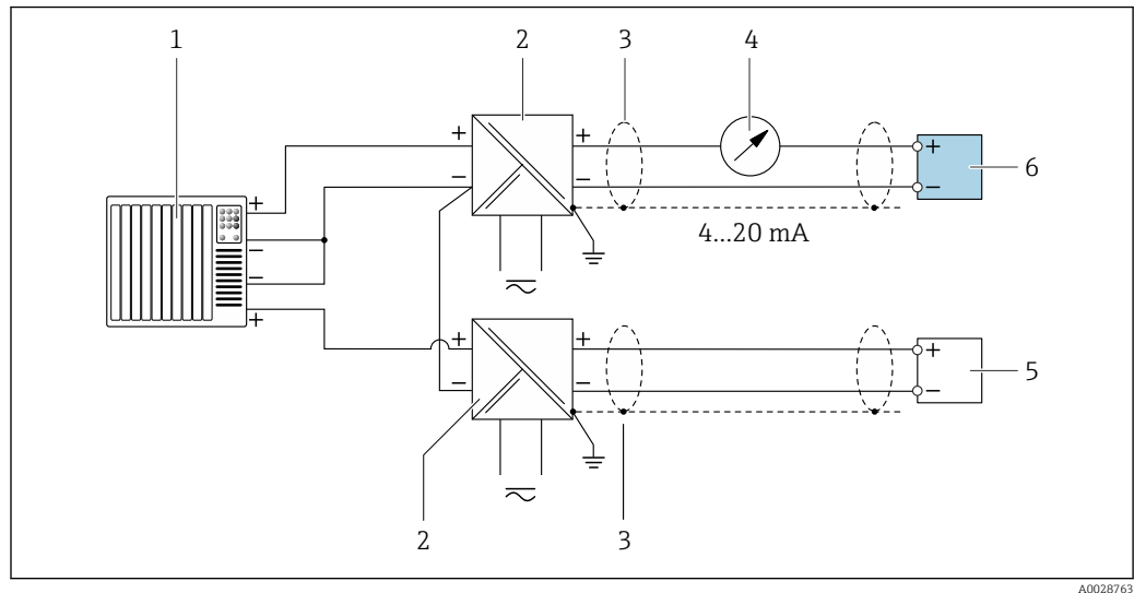
11 Anschlussbeispiel für HART-Eingang mit gemeinsamem "Minus" (passiv)
