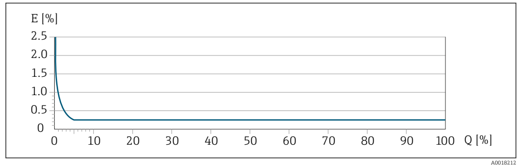
E Maximale Messabweichung in % v.M. (Beispiel: DN 25) Q Durchflussrate in % vom maximalen Endwert
