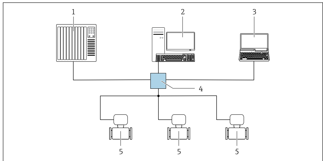
24 Möglichkeiten der Fernbedienung via EtherNet/IP-Netzwerk: Sterntopologie
