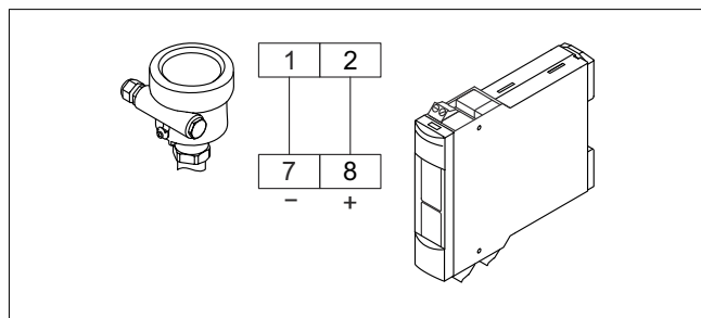
3 Anschluss Messaufnehmer mit Nivotester
