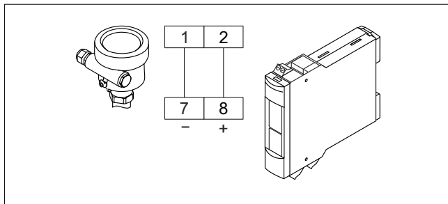
3 Priključivanje senzora na Nivotester
