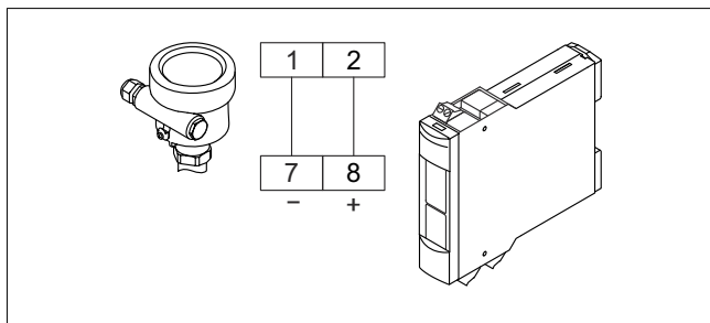
3 Ansluta sensorn till Nivotester
