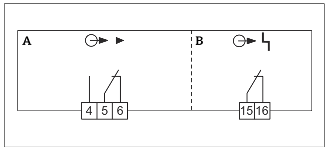
図4 出力の接続
