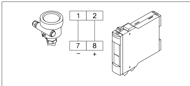
図3 センサと Nivotester の接続
