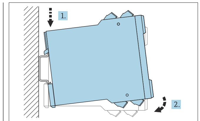
☐ 1 설치; EN 60715 TH35-7.5/EN 60715 TH35-15에 따른 DIN 레일
