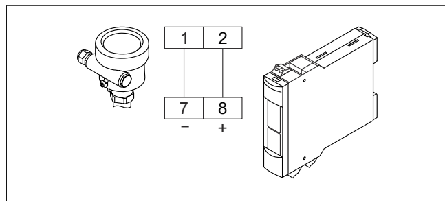
3 Priključitev senzorja na napravo Nivotester
