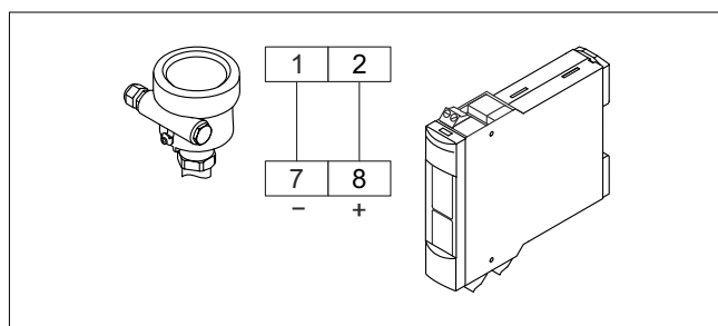
3 Aansluiten van de sensor op de Nivotester
