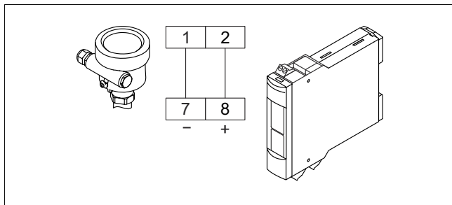
3 Conexão do sensor para o Nivotester
