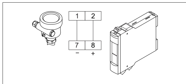
3 Připojení senzoru k Nivotester
