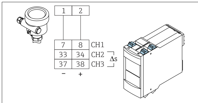
3 Sensörün Nivotestere bağlanması
