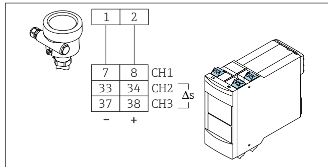
3 Podłączenie sygnalizatora do modułu Nivotester
