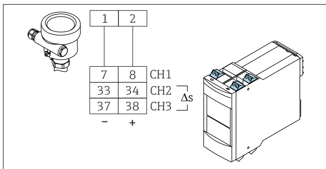
3 Anturin kytkeminen Nivotesteriin
