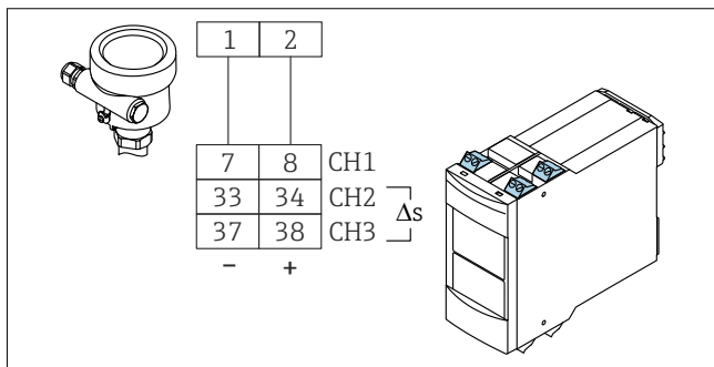
図 3 センサと Nivotester の接続
