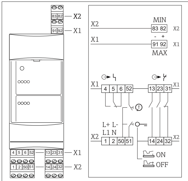
図 2 前面パネル開放、端子台への接続
