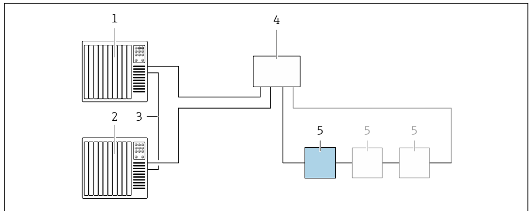
14 Anschlussbeispiel Systemredundanz S2
