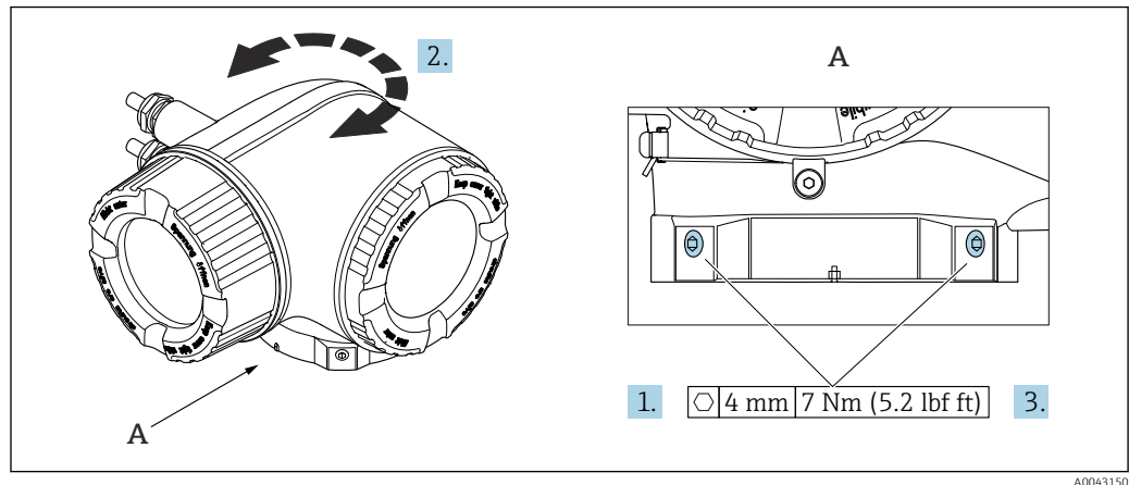
11 Ex-Gehäuse
