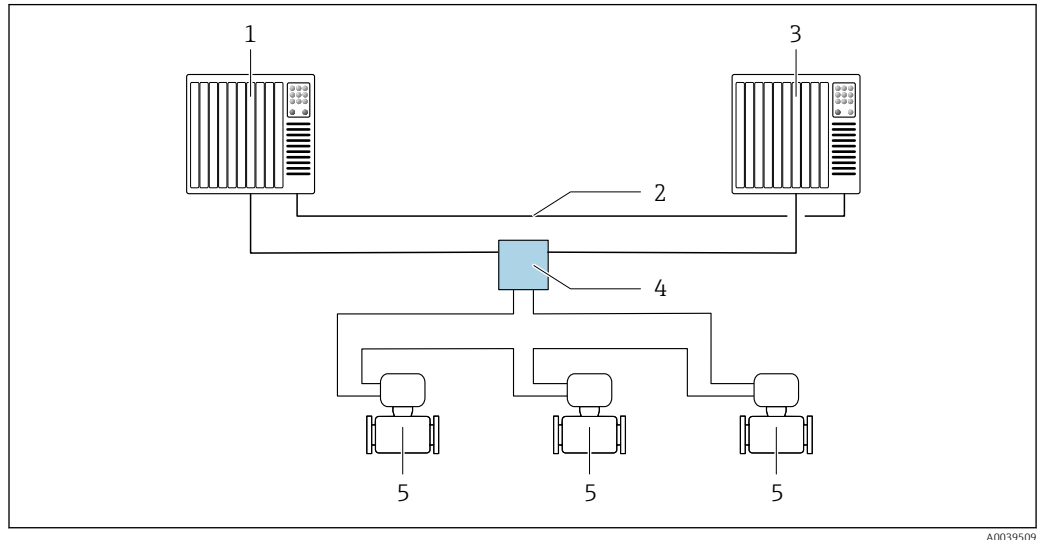
29 Beispiel für den Aufbau eines redundanten Systems (S2): Ringtopologie
