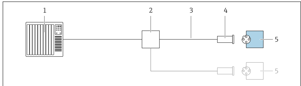
13 Anschlussbeispiel für PROFINET
