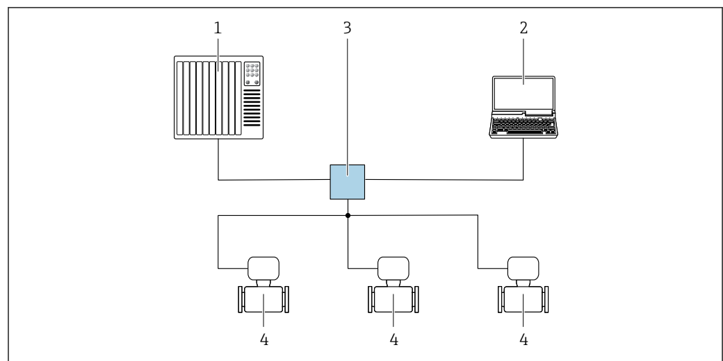
📄 26 Möglichkeiten der Fernbedienung via PROFINET Netzwerk: Sterntopologie
