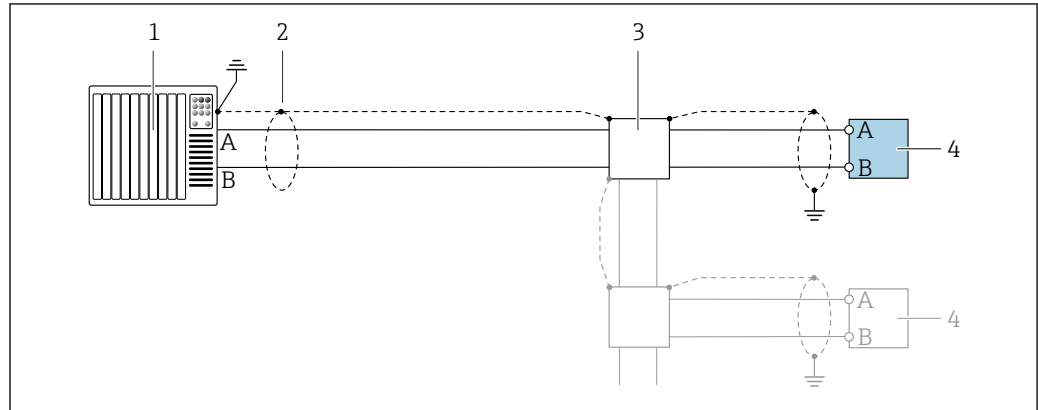
11 Anschlussbeispiel für PROFIBUS DP, nicht explosionsgefährdeter Bereich und Zone 2/Div. 2
