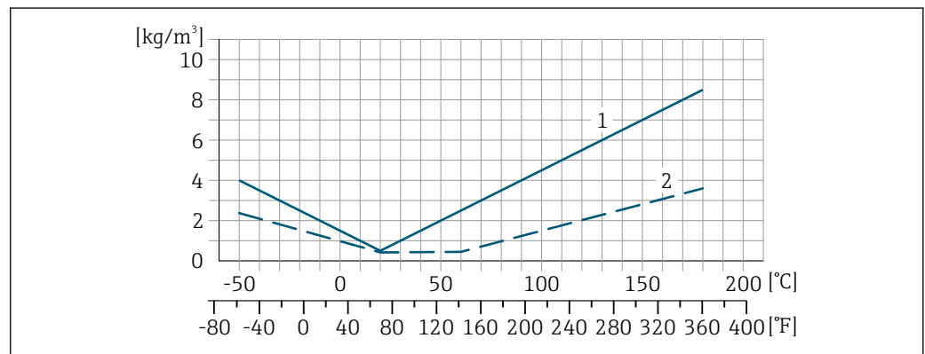
1 Felddichtejustierung, Beispiel bei +20 °C (+68 °F) 2 Erweiterte Dichtekalibrierung
