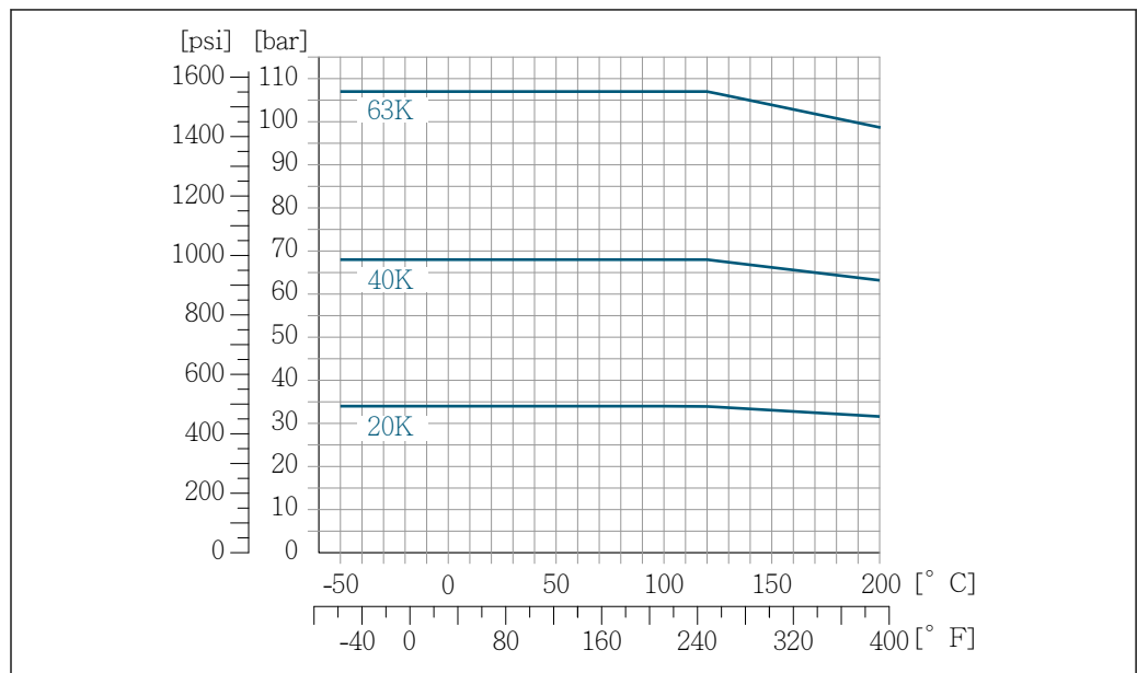
14 Mit Flanschwerkstoff: 1.4404 (316/316L) oder Alloy C22, 2.4602 (UNS N06022)
