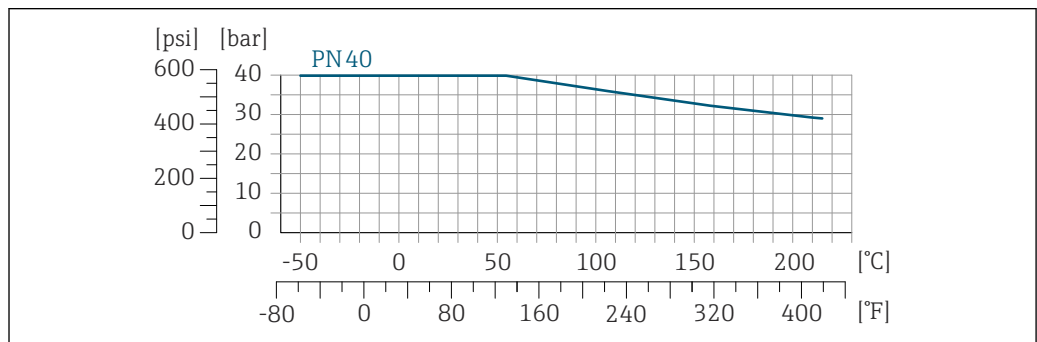
10 Losflansch mit Flanschwerkstoff: 1.4301 (F304), mediumsberührende Teile Alloy C22: 2.4602 (UNS N06022)
