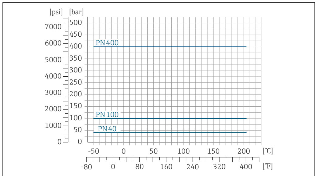
9 Mit Flanschwerkstoff: Alloy C22, 2.4602 (UNS N06022)
