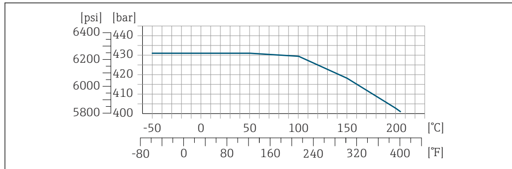
18 Mit Flanschwerkstoff: Alloy C22, 2.4602 (UNS N06022); Bestellmerkmal "Messrohr Mat., Oberfläche mediumberührt", Option HB
