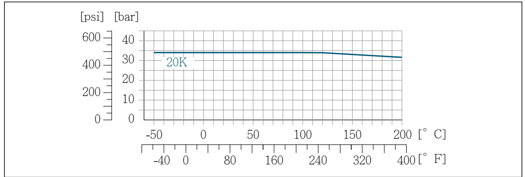
15 Losflansch mit Flanschwerkstoff: 1.4301 (F304), mediumsberührende Teile Alloy C22: 2.4602 (UNS N06022)
