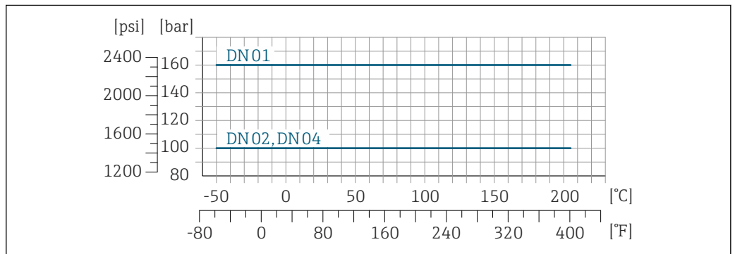
16 Mit Flanschwerkstoff: 1.4404 (316/316L)
