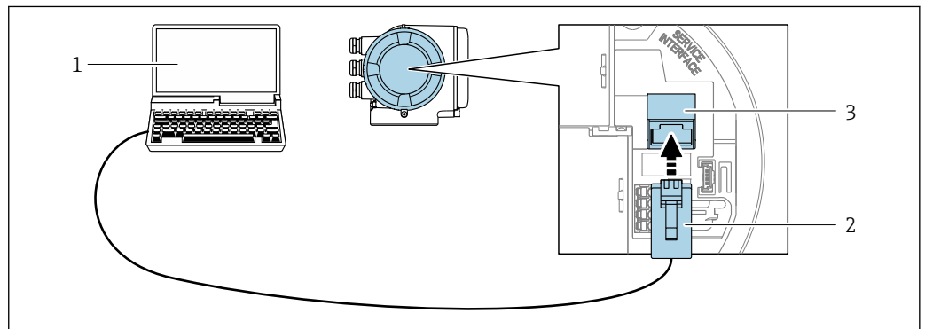
☐ 36 サービスインタフェース (CDI-RJ45) 経由の接続
