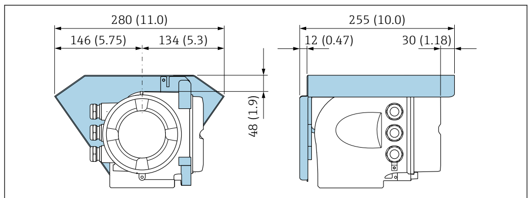
図 12 Proline 500 用の日除けカバー、工学単位 mm (in)
