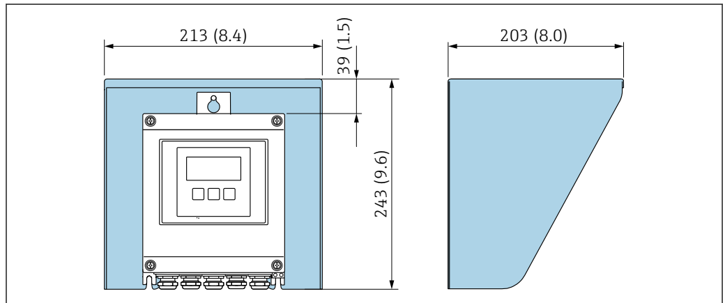
図 11 Proline 500 – デジタル用の日除けカバー、工学単位 mm (in)
