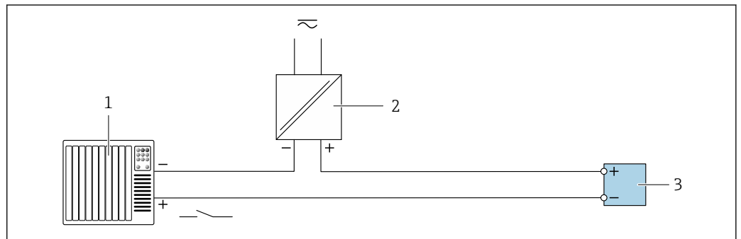
图 31 接线实例：状态输入
