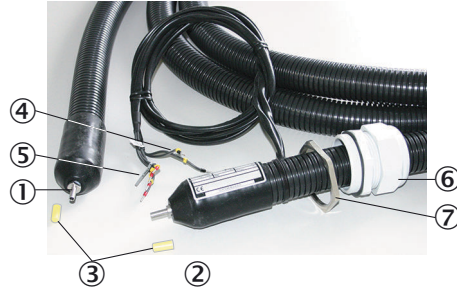
Abbildung 4: Beheizte Messgasleitung
