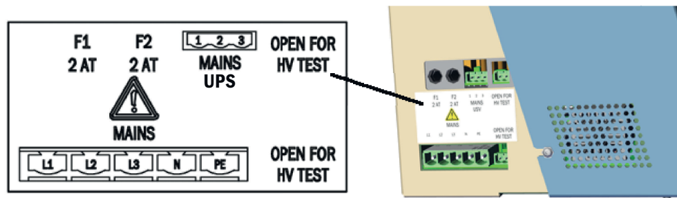
Abbildung 13: Anschluss Spannungsversorgung
