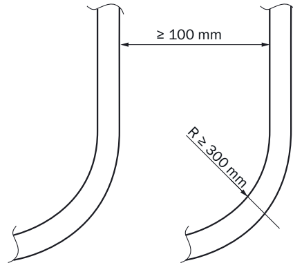
Abbildung 11: Leitungen – Abstand und Biegeradius
