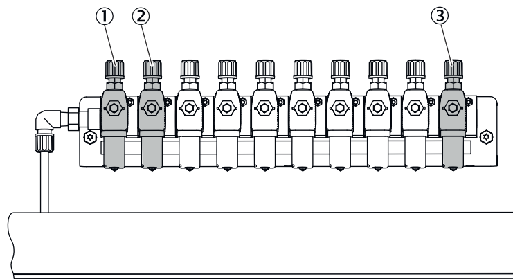
Abbildung 12: Anschlüsse der Prüfgaseinheit
