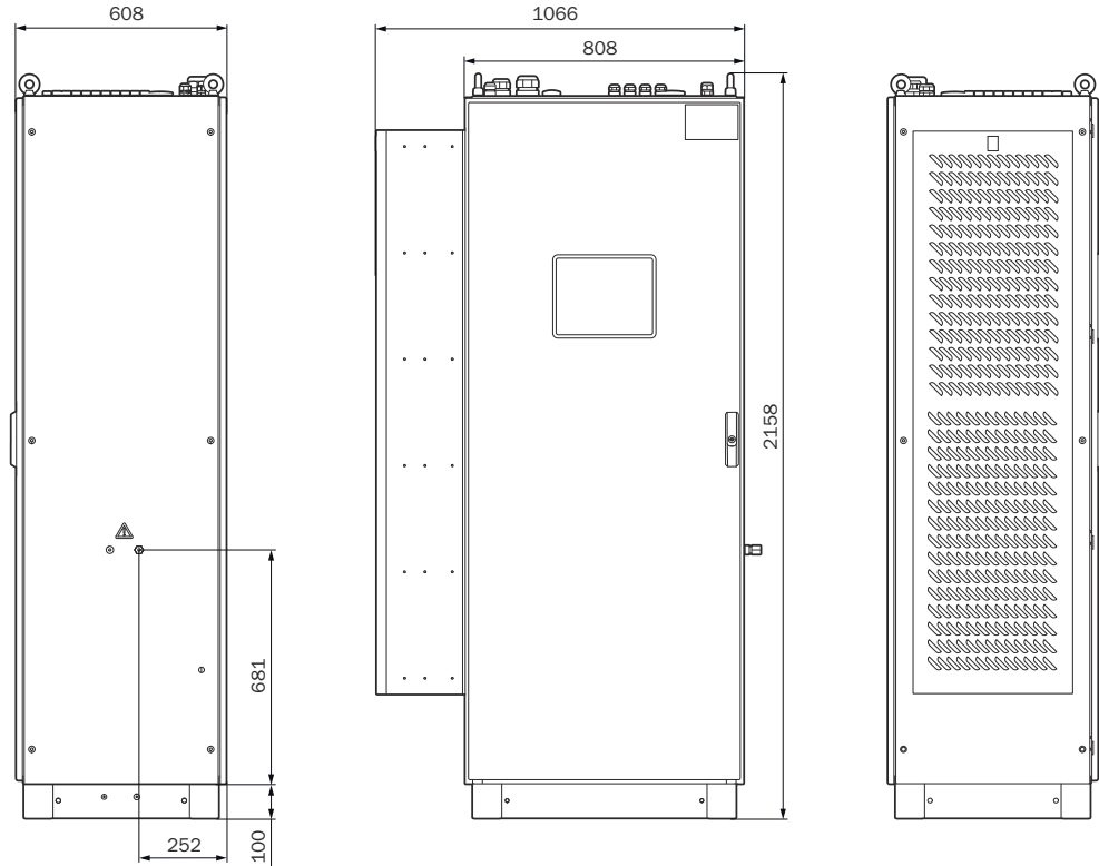
Abbildung 23: Maßzeichnung MCS200HW in Edelstahl
