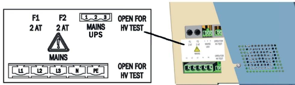
Abbildung 14: Anschlüsse Spannungsversorgung
