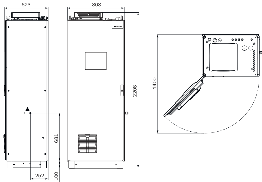
Abbildung 21: Maßzeichnung MCS200HW in Grundkonfiguration
