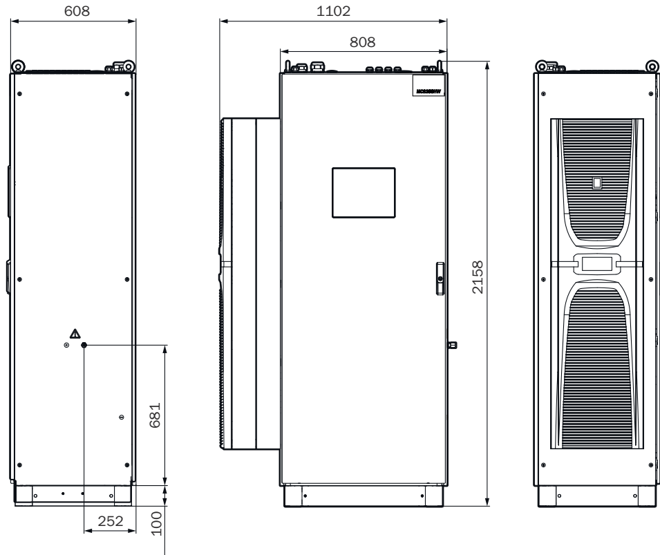
Abbildung 22: Maßzeichnung MCS200HW mit Kühlgerät
