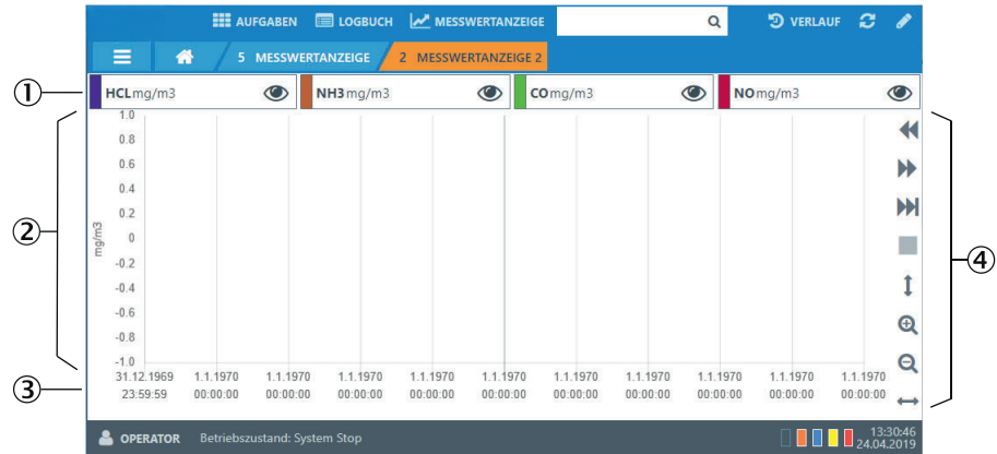
Abbildung 17: Messwertanzeige
