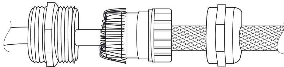
Abbildung 15: Anschlüsse Signalleitungen (abgeschirmt)
