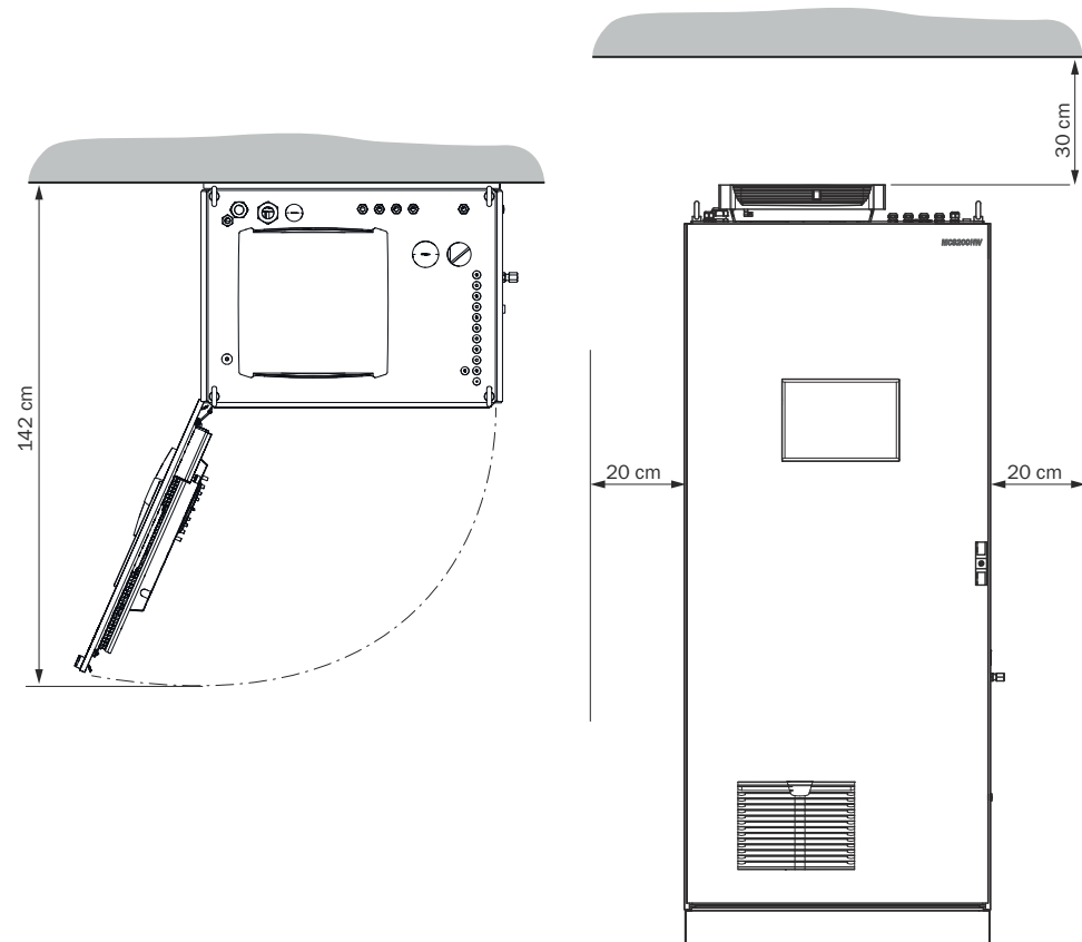
Abbildung 6: Darstellung für Grundkonfiguration
