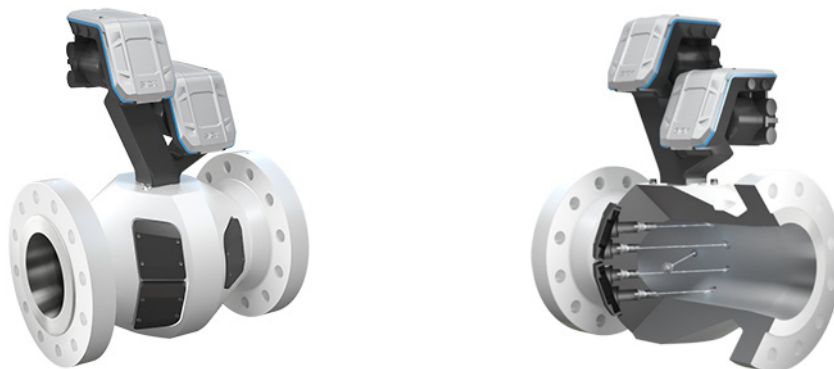
图 6 FLOWSIC600-XT 2plex
