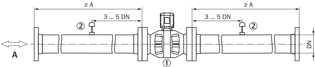
图 22 双向使用，不带整流盘（配置 A）
