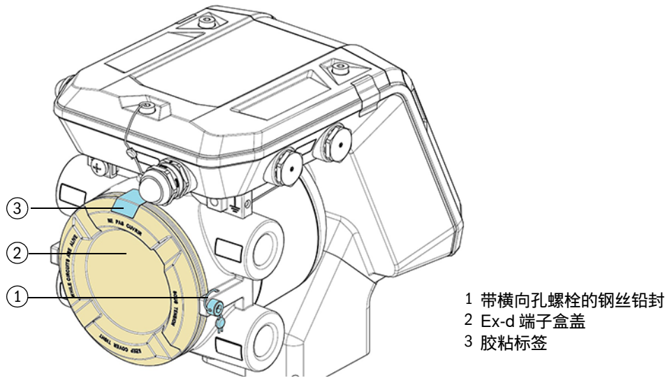
图 18 Ex-d 端子盒的封装
