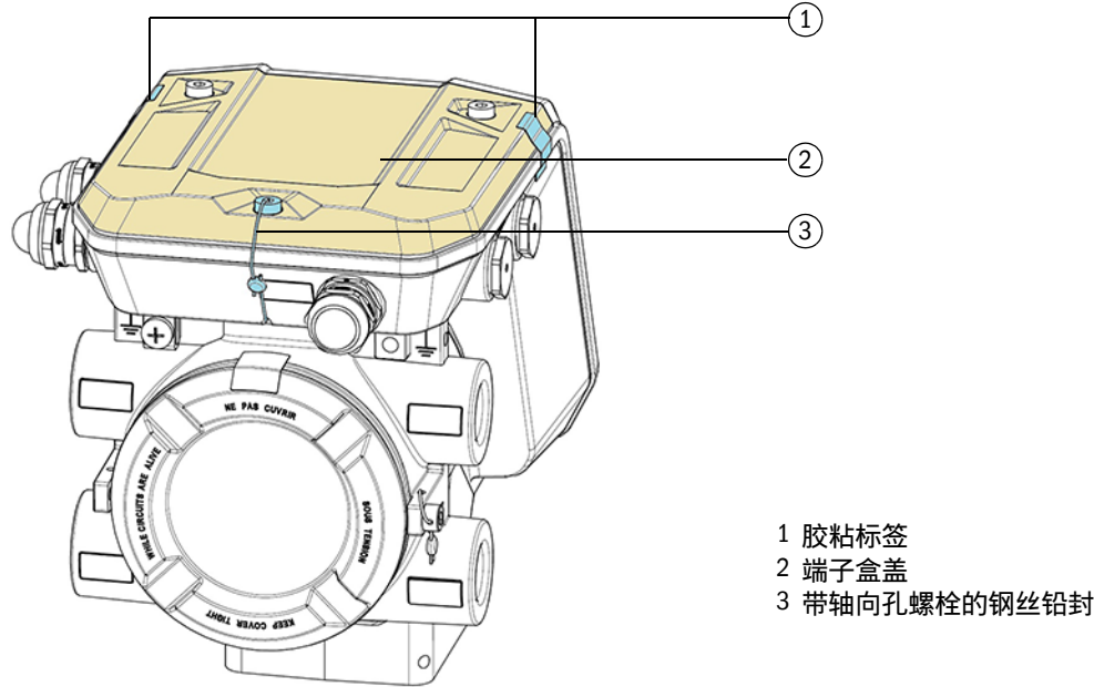
图 19 Ex-e 或 Ex-i 端子盒的封装
