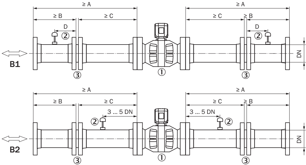
图 23 双向使用，带整流盘（配置 B）
