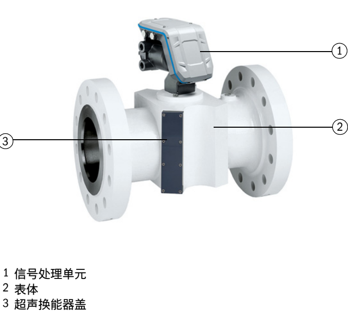
图 3 FLOWSIC600-XT C 概览
