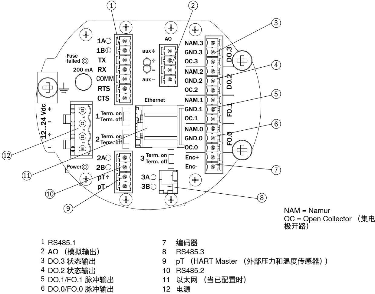
图 35 Ex-d 端子盒的端子布置
