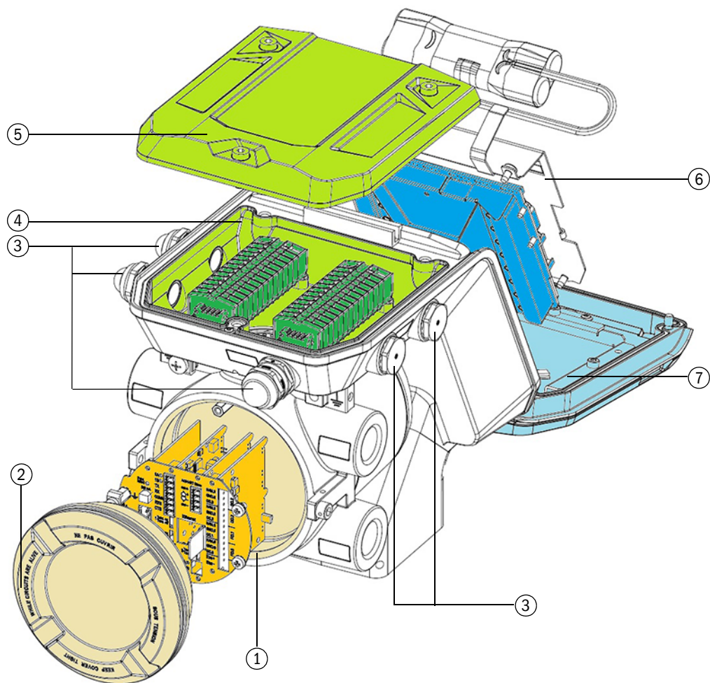
图 32 外壳种类 Ex-de
