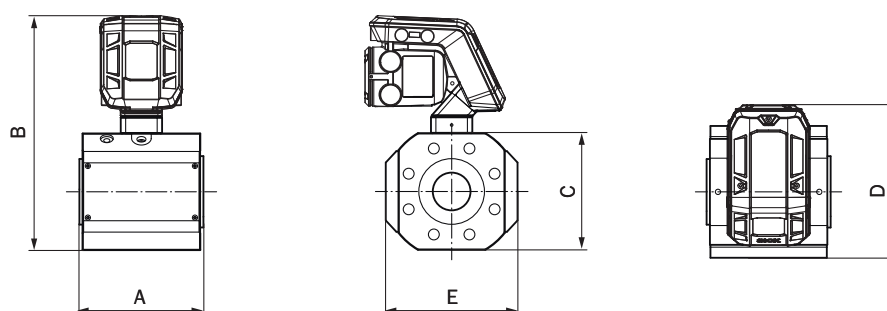
图 65 FLOWSIC600-XT: 3" 结构, 压力等级最大到 Class 600/PN100
