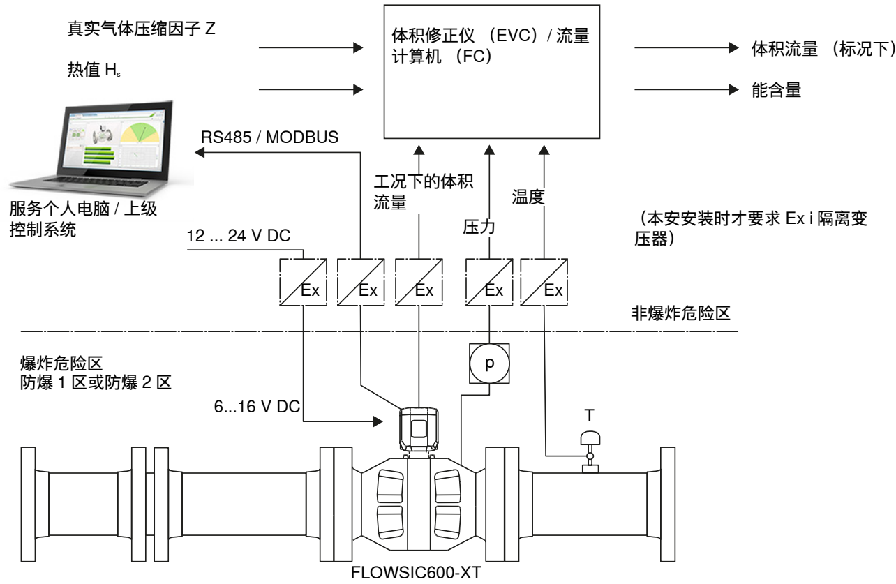
图 30 FLOW SIC600-XT 接线图
