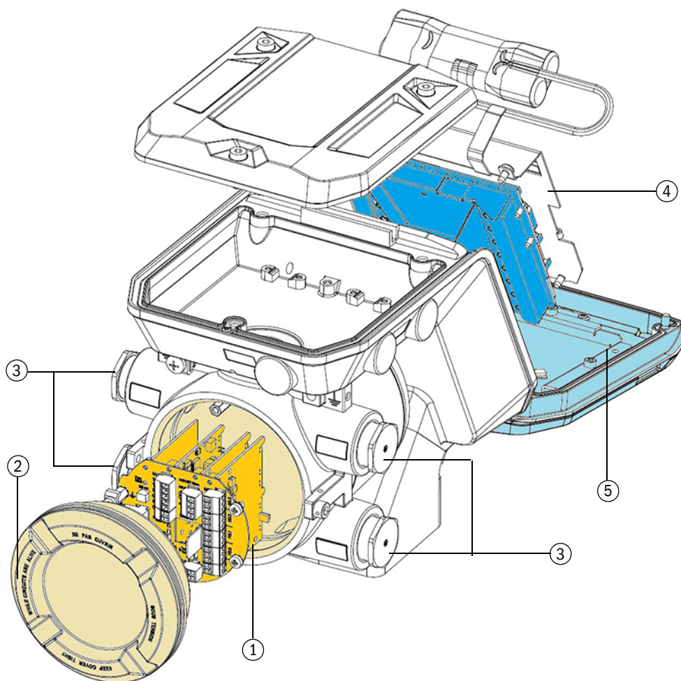
图 31 外壳种类 Ex-d
