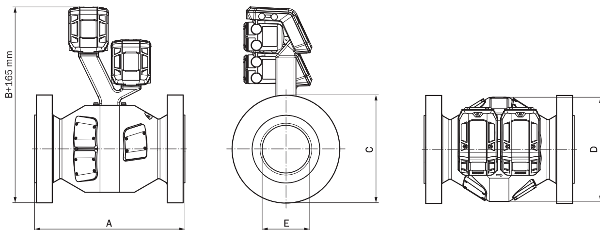
图 64 FLOWSIC600-XT 2plex 和 FLOWSIC600-XT Quatro
