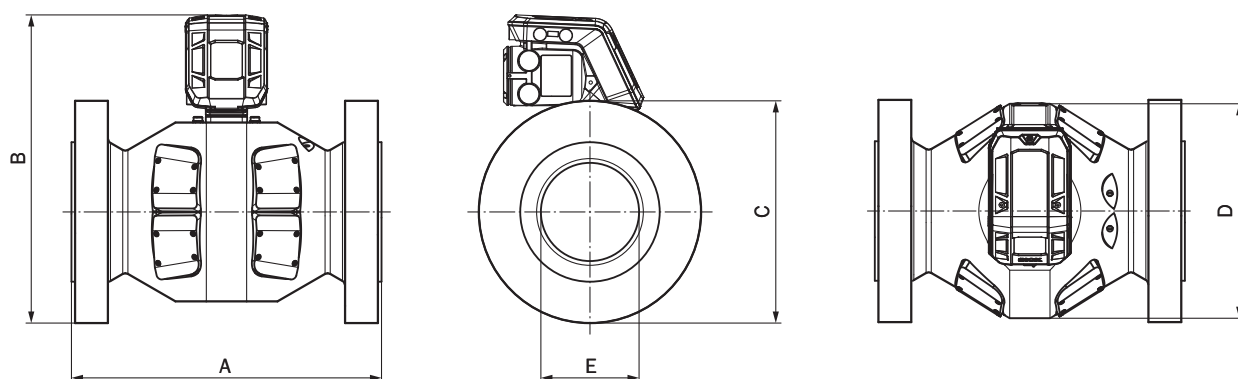
图 63 FLOWSIC600-XT 和 FLOWSIC600-XT Forte
