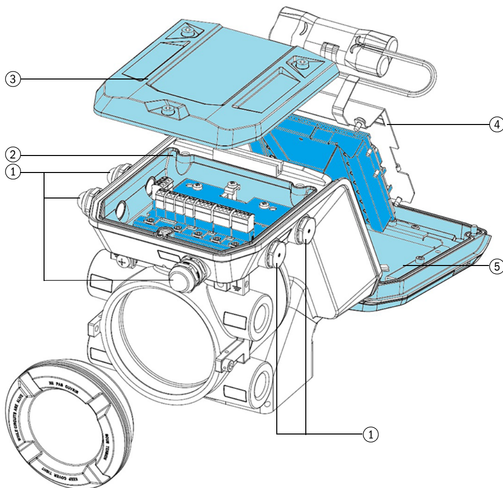
图 33 外壳种类 Ex-i
