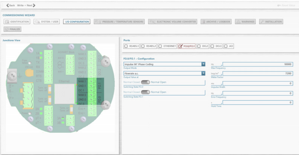
图 43 配置输入 / 输出 (I/O configuration)
