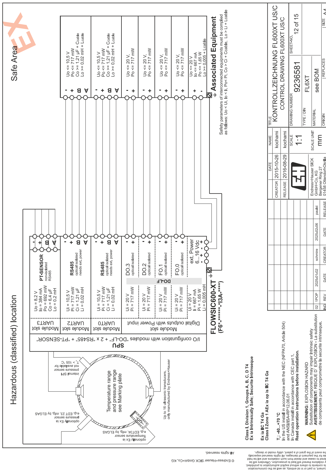
图 81 接线图 9236581 (第 12 页)
