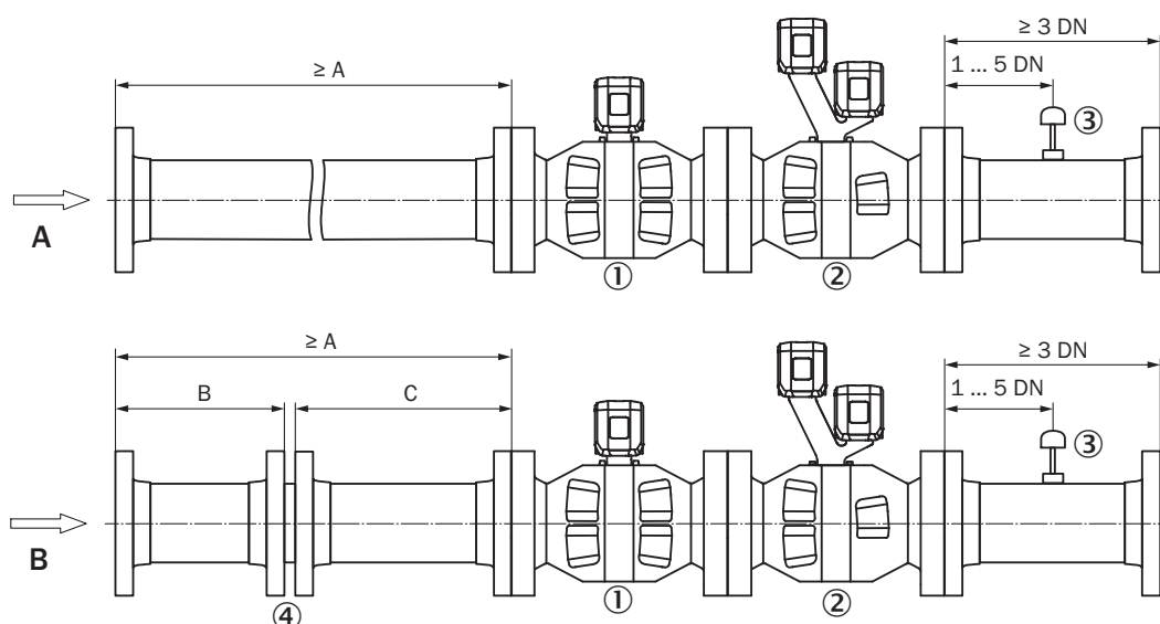
单向法兰 - 法兰安装
