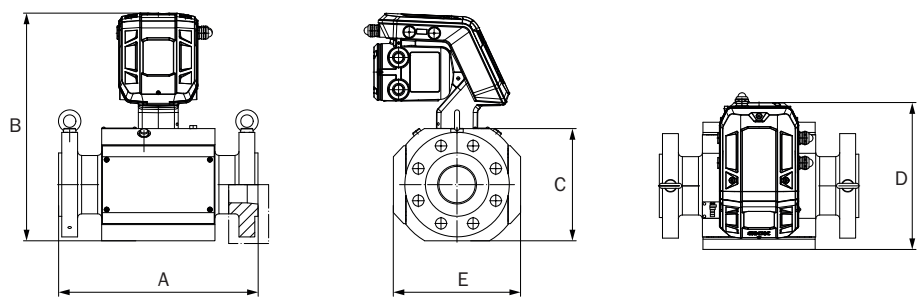
图 66 FLOWSIC600-XT: 3" - 5D 结构
