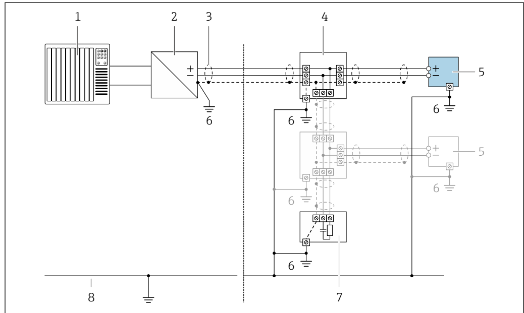
图 12 PROFIBUS PA 的接线实例
