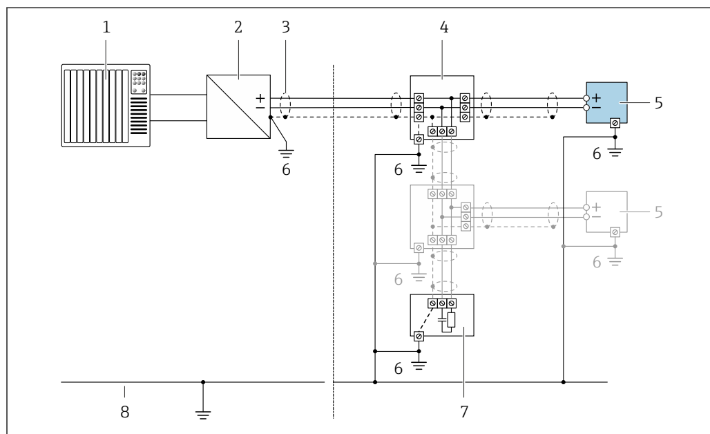
12 Exemplo de conexão para PROFIBUS PA
