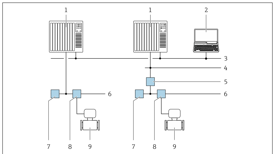
26 Opzioni per il funzionamento a distanza mediante rete FOUNDATION Fieldbus
