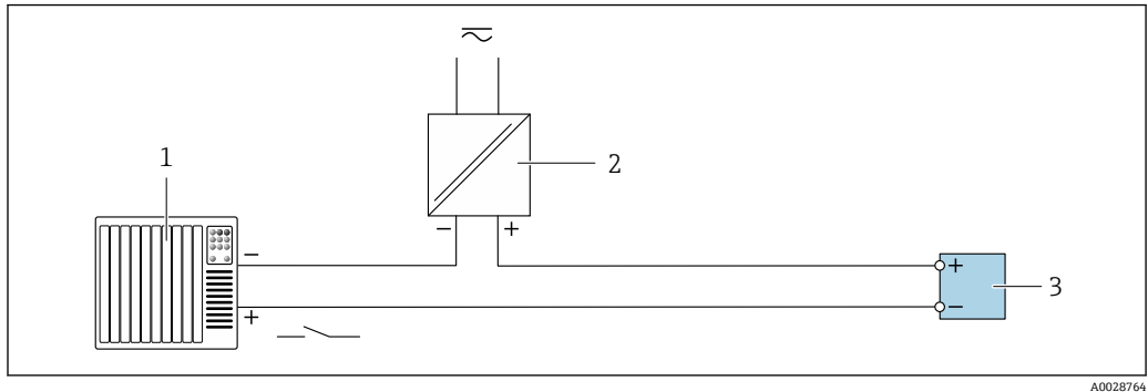
图 22 接线实例：状态输入
