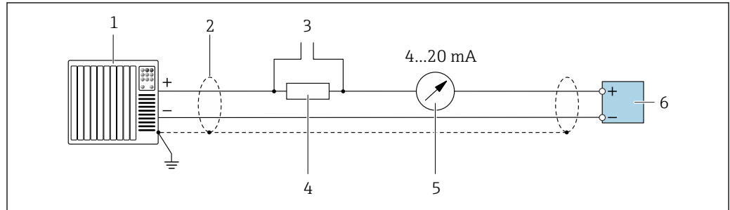
图 11 4...20 mA HART 电流输出 (有源) 的接线图
