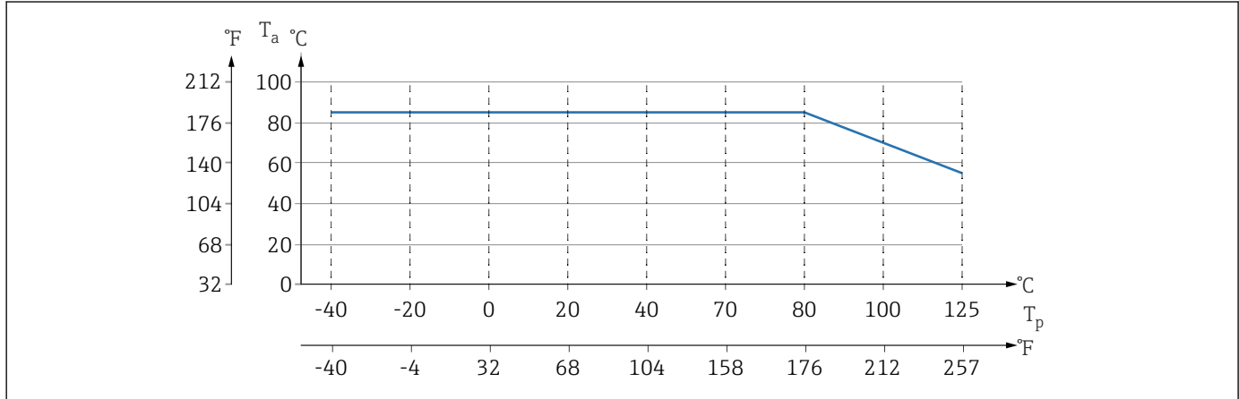
图 12 以上为无保温层垂直安装时的温度范围。
