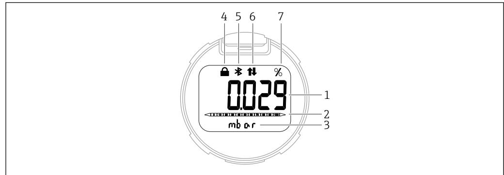
图 4 段码显示屏
