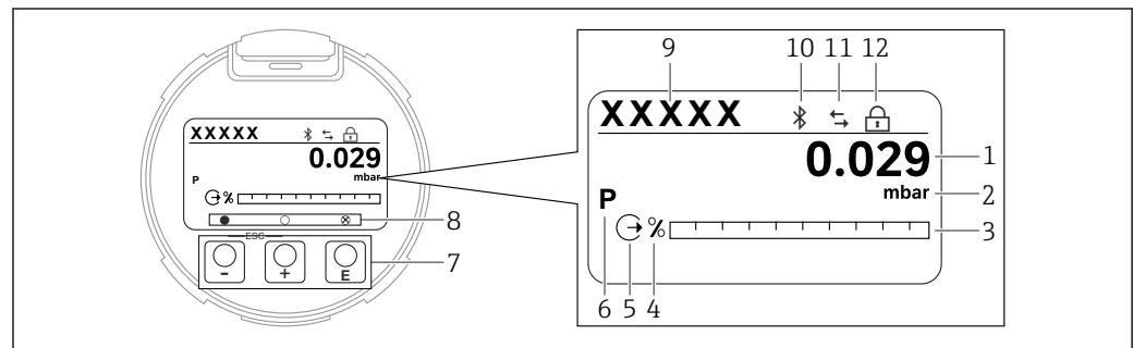
图 5 图形显示屏, 带光敏键。
