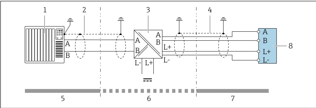
15 接线实例：本安 Modbus RS485
