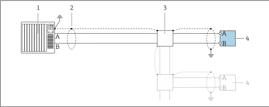
14 接线实例，Modbus RS485，非防爆危险区和 Zone 2 / Div. 2 防爆危险区
