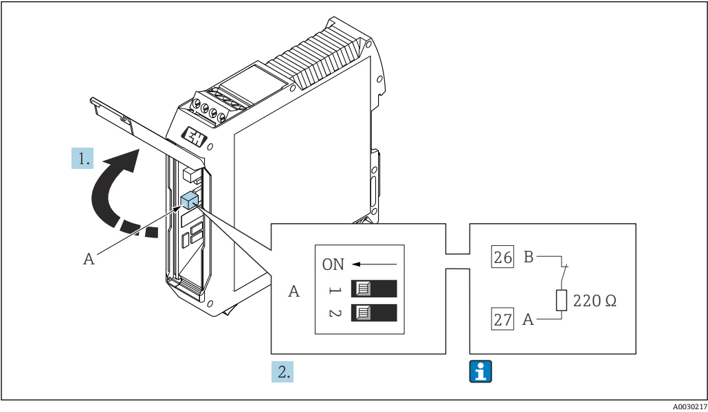
图 17 通过 Promass 100 安全栅上的 DIP 开关开启终端电阻
