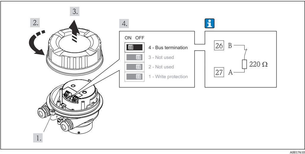
图 16 通过电子模块上的 DIP 开关开启终端电阻
