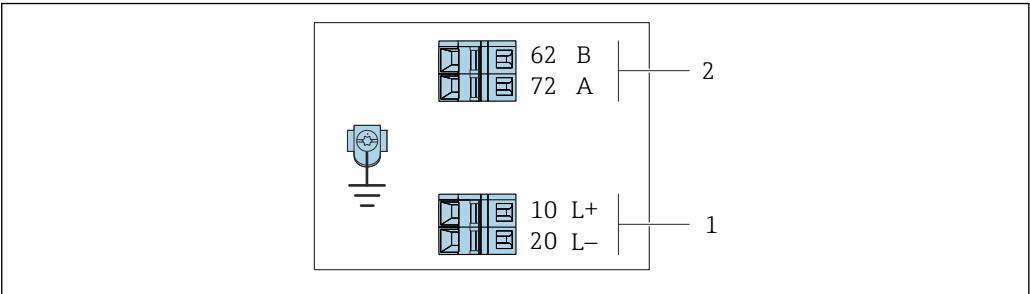
9 接线端子分配: Modbus RS485, 在本安防爆区中使用 (通过 Promass 100 安全栅连接)
