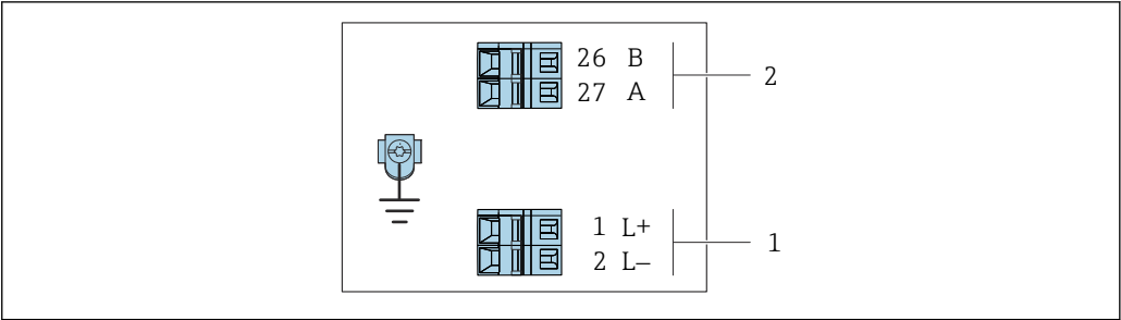
8 Modbus RS485 接线端子分配，连接类型适用非危险区和 Zone 2/ Div. 2 防爆场合
