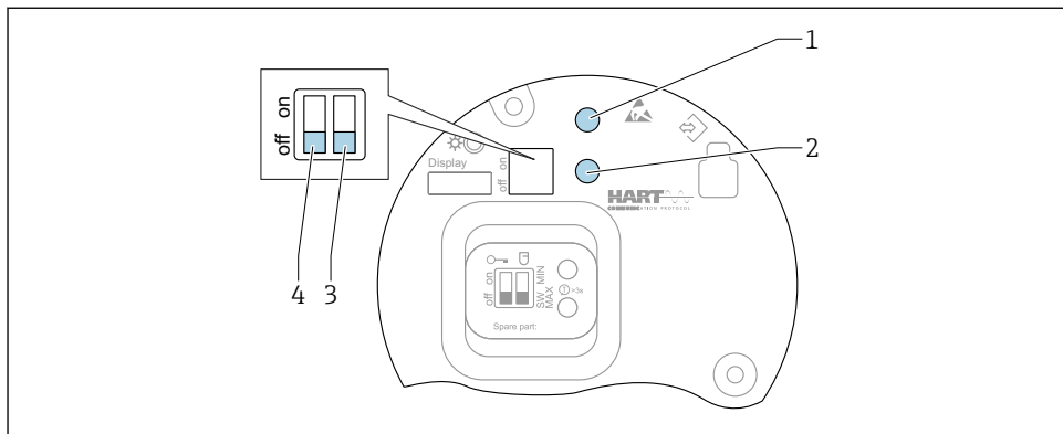
15 Touches de configuration et commutateurs DIP sur l'électronique HART
