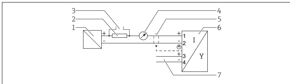
4 Funkční schéma 4 ... 20 mA HART, spínací výstup
