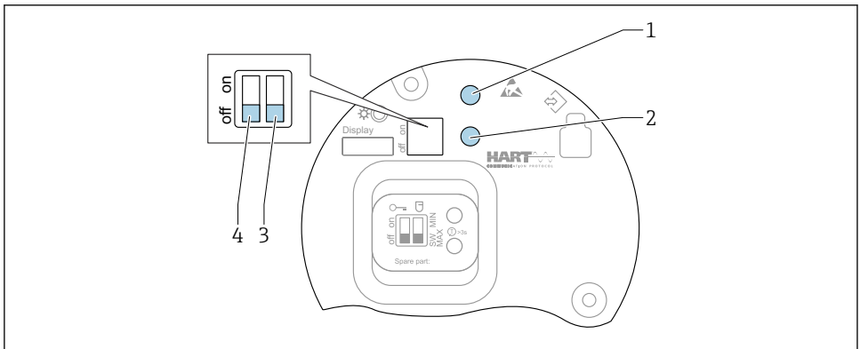
15 Bedientasten und DIP-Schalter auf dem HART Elektronikeinsatz
