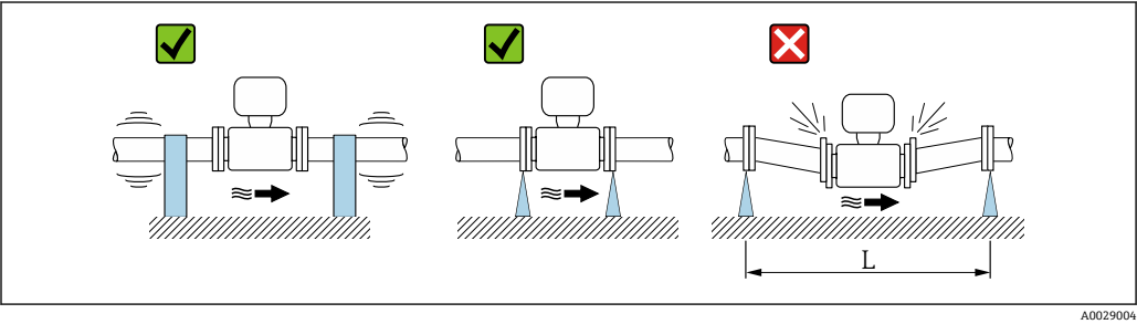
图 7 避免仪表振动的措施 (L > 10 m (33 ft))
