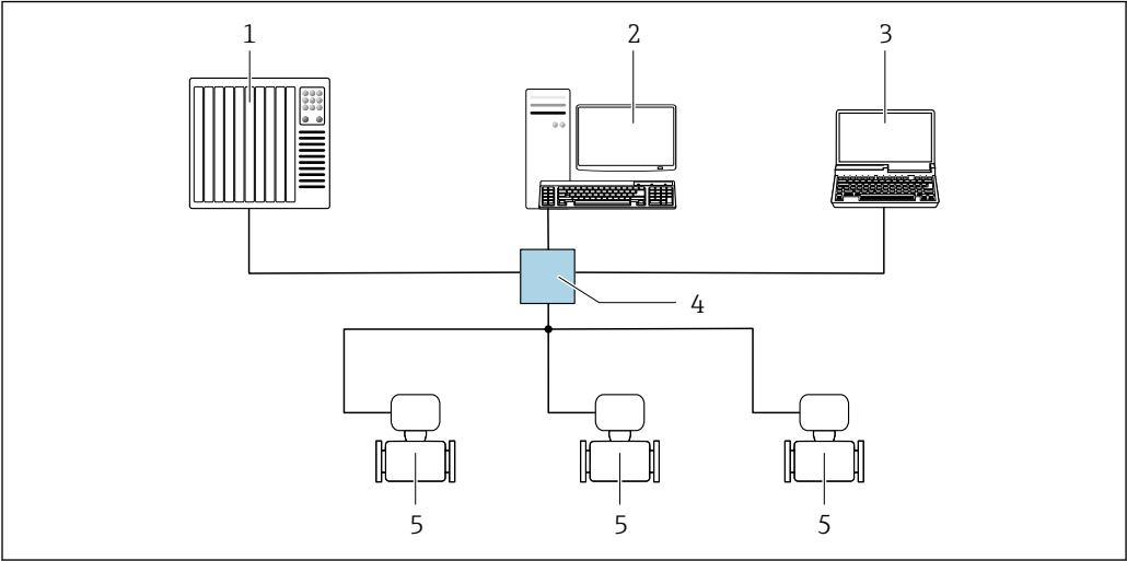
19 通过 EtherNet/IP 网络实现远程操作：星形拓扑结构
