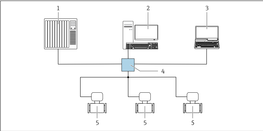
图 14 通过 EtherNet/IP 网络实现远程操作：星形拓扑结构
