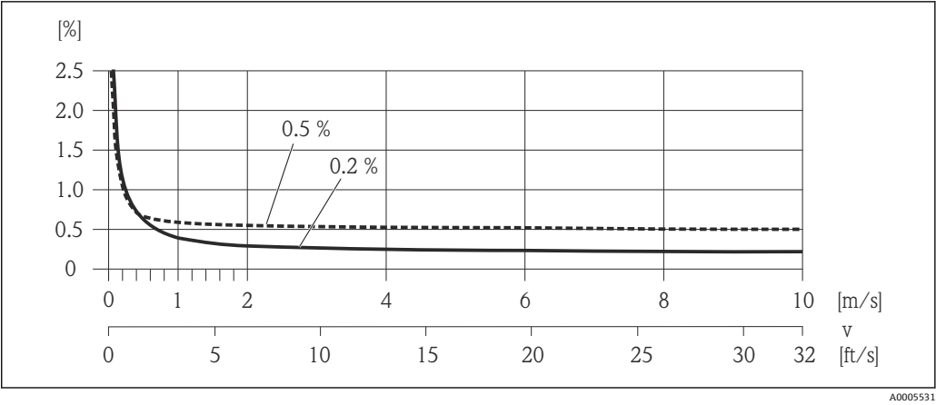
16 最大测量误差 (% o.r.)
