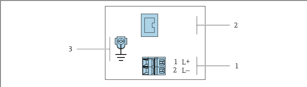
8 EtherNet/IP 型仪表的接线端子分配
