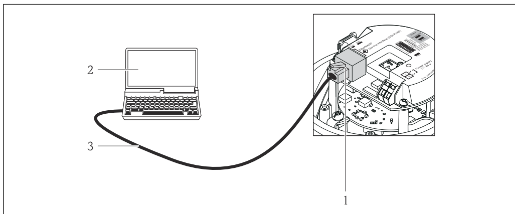
20 Connessione per codice d'ordine per "Uscita", opzione N: EtherNet/IP
