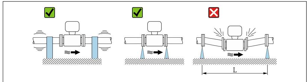
7 Misure per evitare vibrazioni del dispositivo ( L > 10\text{ m} (33 ft))
