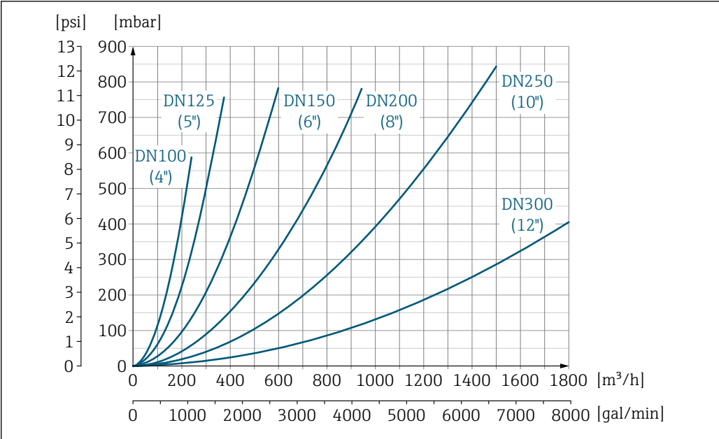
图 19 DN 100...300 (4...12")的压损 (订购选项“设计”, 选项代号 C “短插入深度, 符合 ISO/DVGW 标准 (最大适用口径为 DN 300), 测量管不带前后直管段”)
