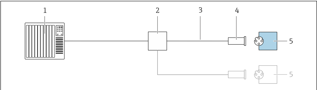
12 接线实例：PROFINET
