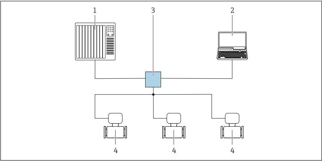
图 20 通过 PROFINET 网络实现远程操作：星形拓扑结构
