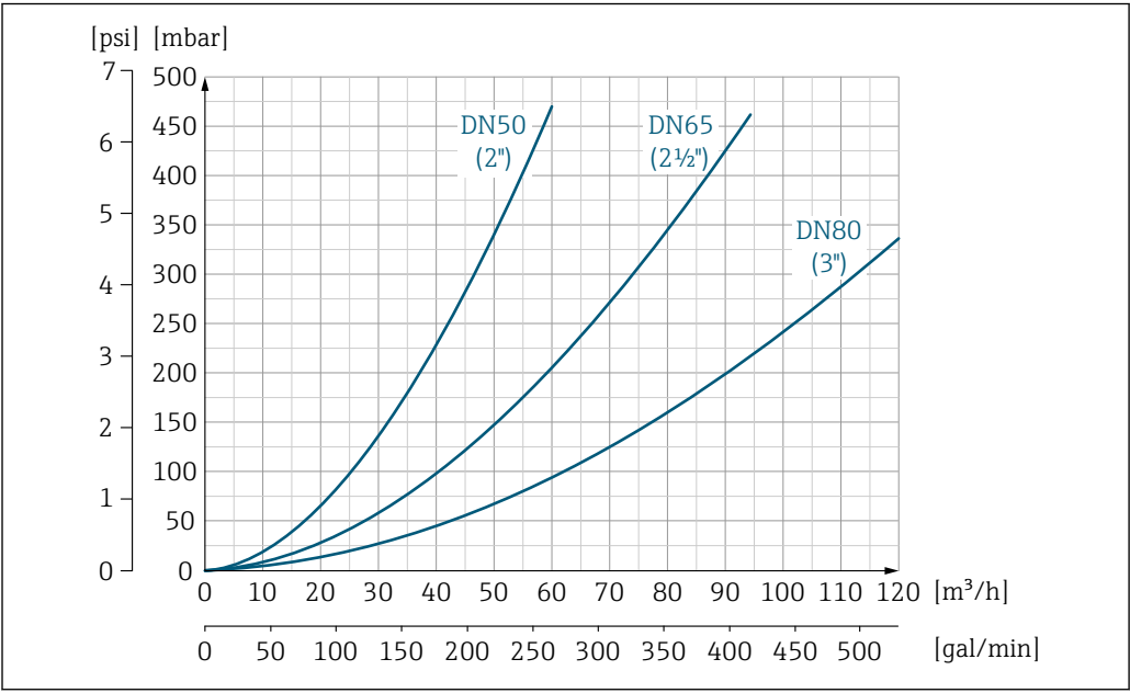
图 18 DN 50...80 (2...3")的压损 ("订购选项"设计", 选项代号 C "短插入深度, 符合 ISO/DVGW 标准 (最大适用口径为 DN 300) , 测量管不带前后直管段")
