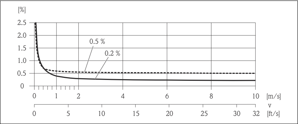
17 最大测量误差 (% o.r.)
