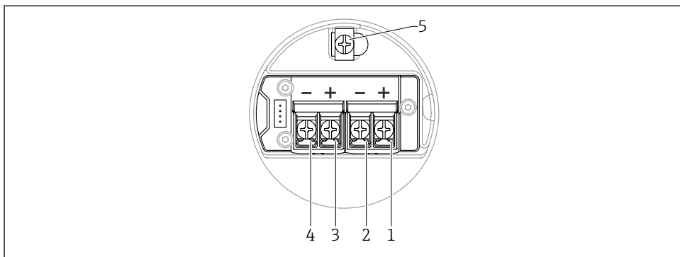
14 Klemmenbelegung im Anschlussraum; 4 ... 20 mA HART, Schaltausgang; Zweikammergehäuse L-Form
