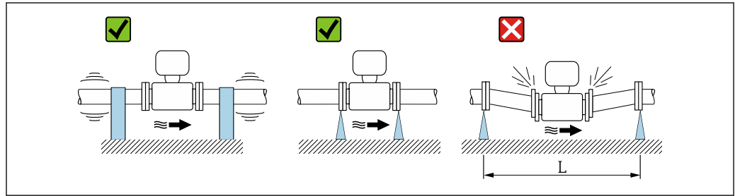
图 7 避免仪表振动的措施 ( L > 10\text{ m} (33 ft))
