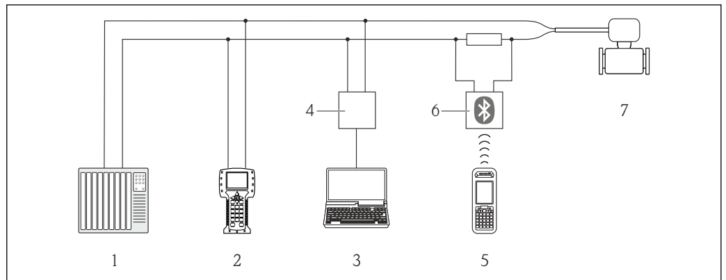
图 19 通过 HART 通信进行远程操作
