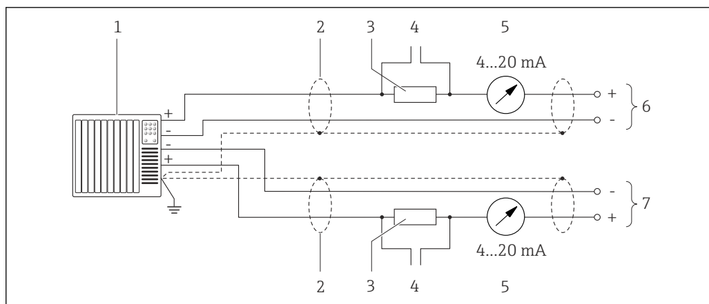
17 Esempio di connessione per l'ingresso HART (modalità di master) mediante l'uscita in corrente (attiva)
