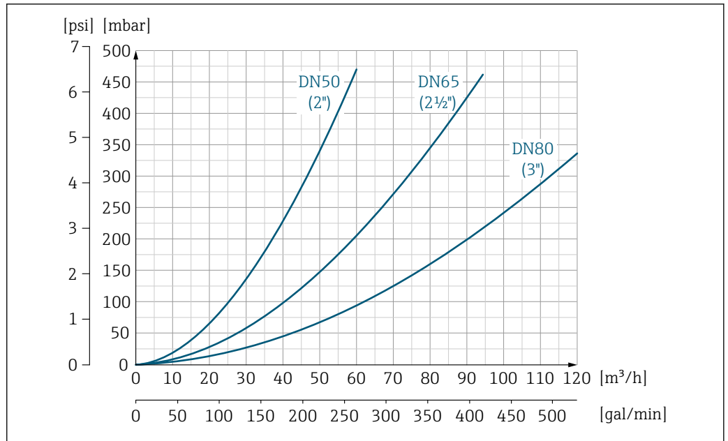
22 Perdita di carico da DN 50 a 80 (da 2 a 3") in caso di codice d'ordine per "Struttura", opzione C "Lunghezza dell'inserzione corta da ISO/DVGW a DN300, senza tratti rettilinei in entrata e in uscita, tubo di misura ristretto"
