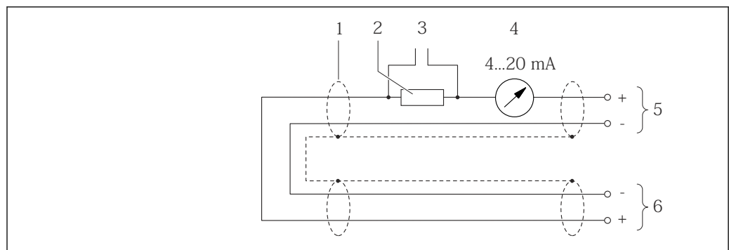
16 Esempio di connessione per l'ingresso HART (modalità di burst) mediante l'uscita in corrente (attiva)
