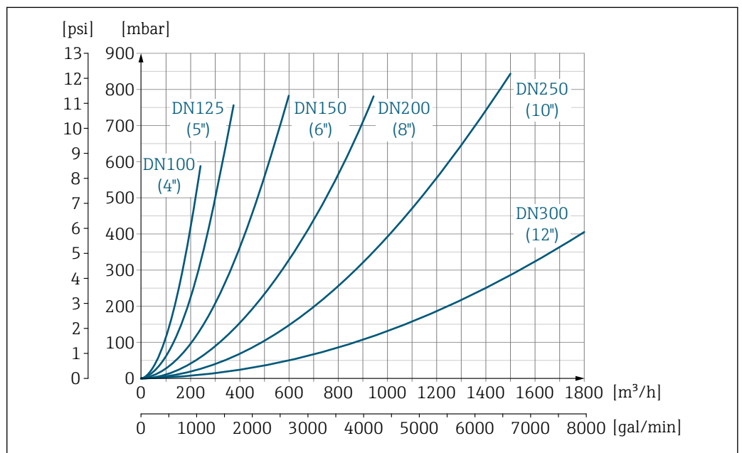
23 Perdita di carico da DN 100 a 300 (da 4 a 12") in caso di codice d'ordine per "Struttura", opzione C "Lunghezza dell'inserzione corta da ISO/DVGW a DN300, senza tratti rettilinei in entrata e in uscita, tubo di misura ristretto"
