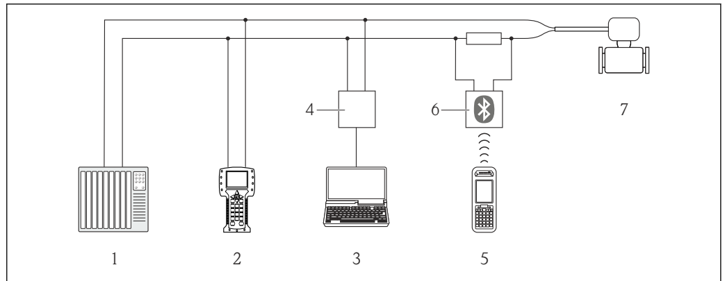
■ 24 Opzioni per il funzionamento a distanza mediante protocollo HART
