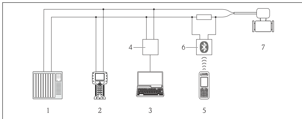
19 Opzioni per il funzionamento a distanza mediante protocollo HART
