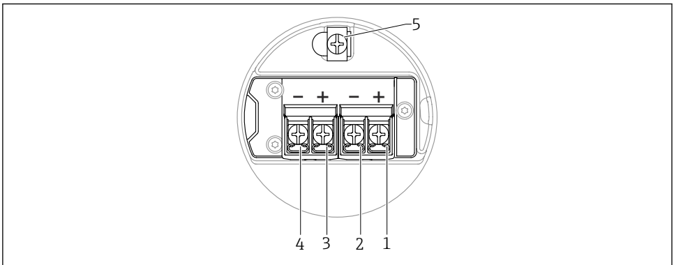
11 Klemmenbelegung im Anschlussraum; 4 ... 20 mA HART, Schaltausgang; Zweikammergehäuse
