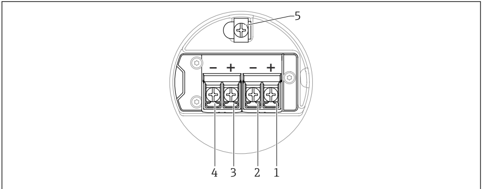
10 Klemmenbelegung im Anschlussraum; 4 ... 20 mA HART + 4 ... 20 mA analog; Zweikammergehäuse
