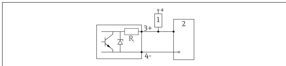
6 Příklad zapojení pro binární vstup
