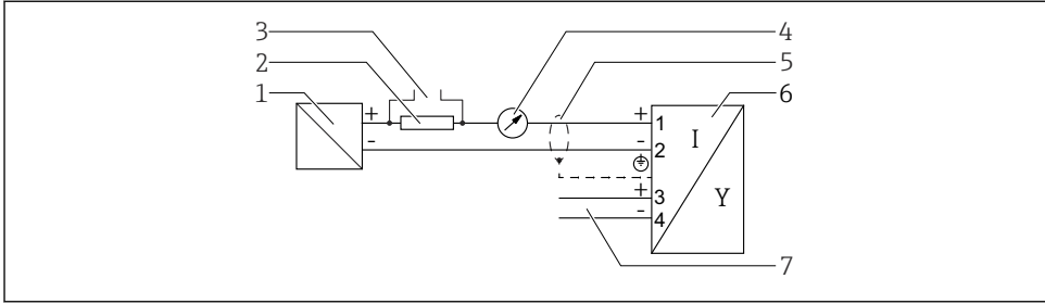
4 Функциональная схема 4 до 20 мА HART, релейный выход
