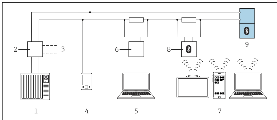
18 Варианты дистанционного управления по протоколу HART
