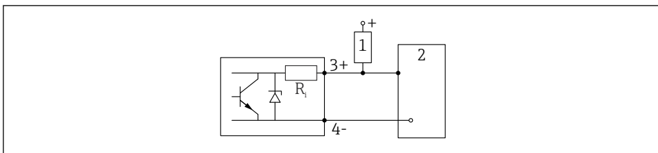
6 Пример подключения через цифровой вход
