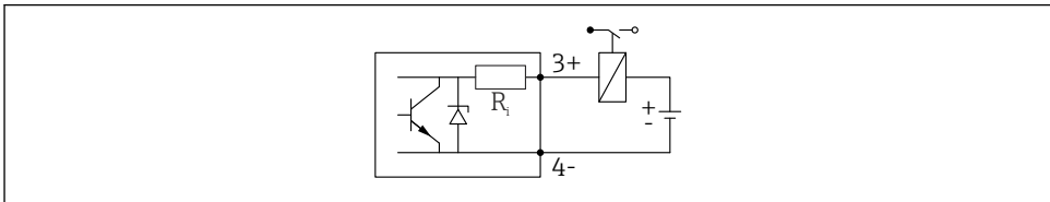
5 Пример подключения реле
