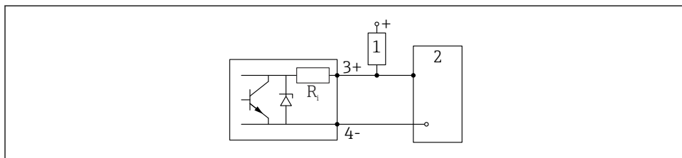
6 Csatlakoztatási példa: digitális bemenet
