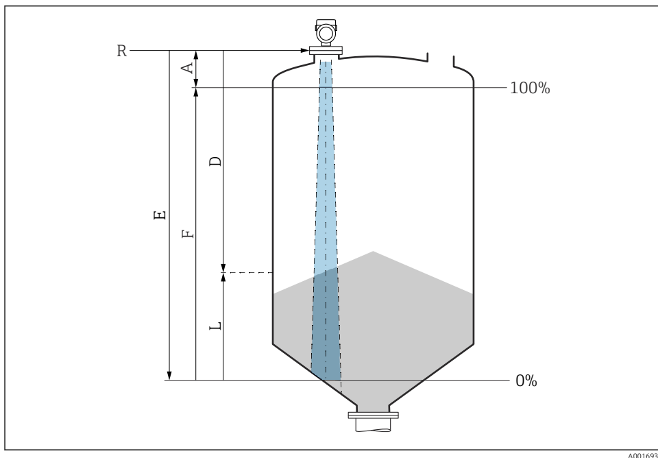
19 Konfigurációs paraméterek ömlesztett szilárd anyagokban történő szintméréshez
