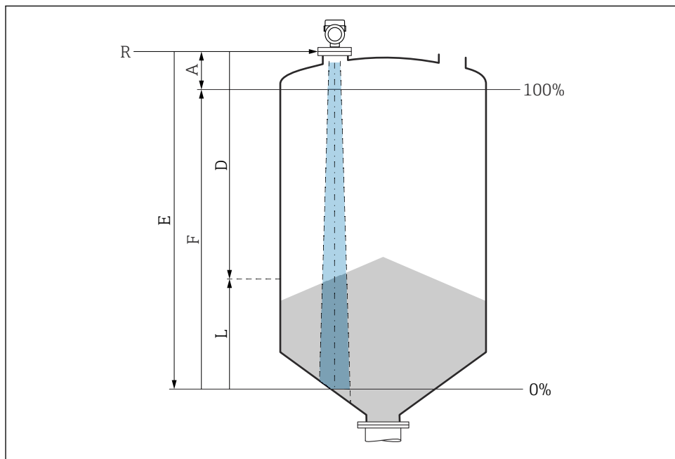
22 Konfigurační parametry pro měření úrovně hladiny v pevných sypkých látkách
