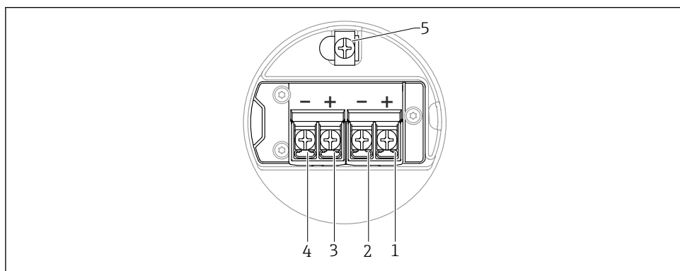
14 Přirazení svorek v připojovacím prostoru; 4 ... 20 mA HART, spínací výstup; dvoukomorové pouzdro
