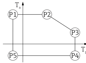
40 Boîtier plastique ; température de process -40 \dots +280 \text{ }^{\circ}\text{C} ( -40 \dots +536 \text{ }^{\circ}\text{F} )
