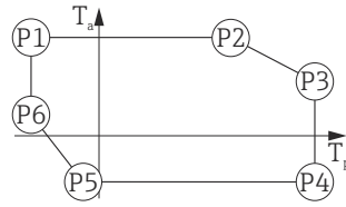
▣ 46 Boîtier plastique ; température de process -196 \dots +200 \text{ }^{\circ}\text{C} ( -320 \dots +392 \text{ }^{\circ}\text{F} )
