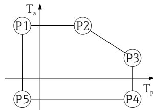
▣ 65 Boîtier 316L, app. hygiénique ; température de process -20 \dots +200 \text{ °C} ( -4 \dots +392 \text{ °F} )
