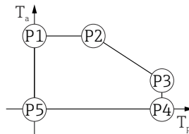
▣ 47 Agrément CSA C/US and boîtier plastique ; température de process 0 \dots +200 \text{ }^{\circ}\text{C} ( +32 \dots +392 \text{ }^{\circ}\text{F} )
