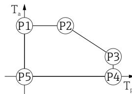
35 Boîtier plastique ; température de process 0 \dots +200 \text{ }^{\circ}\text{C} ( +32 \dots +392 \text{ }^{\circ}\text{F} ) avec agrément CSA C/US
