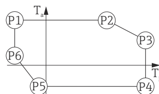
63 Boîtier 316L ; température de process -196 \dots +200 \text{ °C} ( -320 \dots +392 \text{ °F} )
