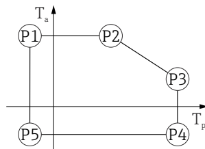
▣ 48 Boîtier alu, revêtu ; température de process -20 \dots +150 \text{ }^{\circ}\text{C} ( -4 \dots +302 \text{ }^{\circ}\text{F} )
