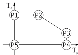
41 Boîtier plastique ; température de process 0 \dots +280 \text{ }^{\circ}\text{C} ( +32 \dots +536 \text{ }^{\circ}\text{F} ) avec agrément CSA C/US
