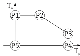
33 Boîtier plastique ; température de process 0 \dots +150 \text{ °C} ( +32 \dots +302 \text{ °F} ) avec agrément CSA C/US
