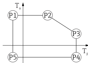
▣ 66 Boîtier 316L, app. hygiénique ; gamme de température de process : -40 \dots +150 \text{ °C} ( -40 \dots +302 \text{ °F} )
