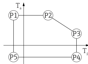
32 Boîtier plastique ; température de process -20 \dots +150 \text{ °C} ( -4 \dots +302 \text{ °F} )
